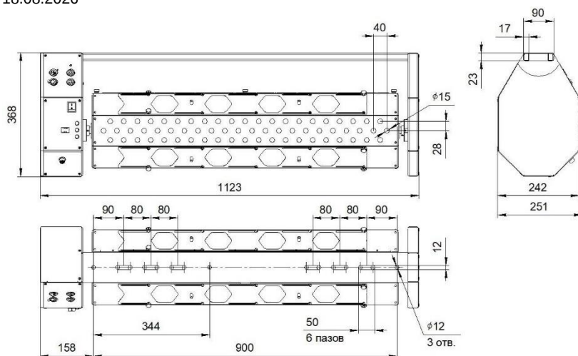
Рисунок. 1 Габаритные размеры
